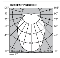
TC-DD 16Вт
