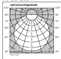
TC-DD 28Вт
