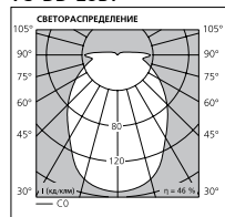
TC-DD 28Вт
