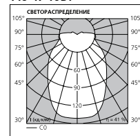
T16-R 40Вт
