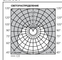
2x58Вт
