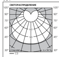
8Вт
