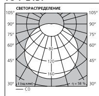
TC-F 24Вт
