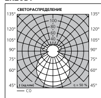
2x26Вт
