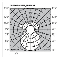
28Вт
