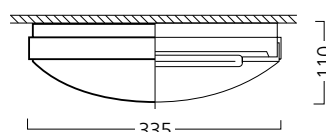
335 Поверхностный
