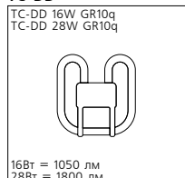
TC-DD
