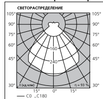
HSL400Вт Призм.акрил
