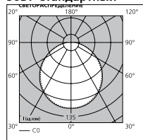
38Вт Стандартный
