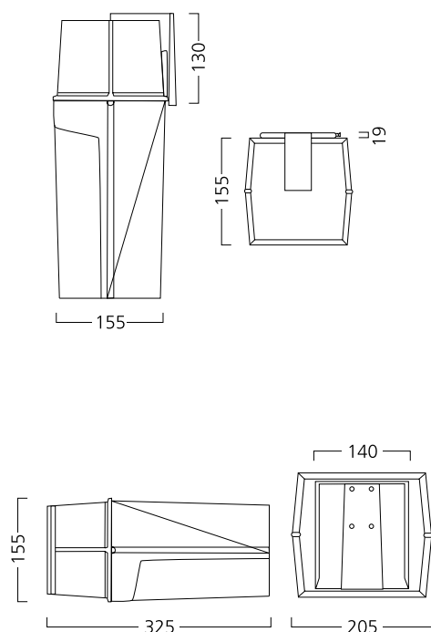
Вертикальный монтаж
