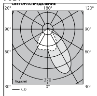
70Вт
