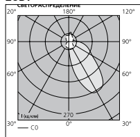
26Вт
