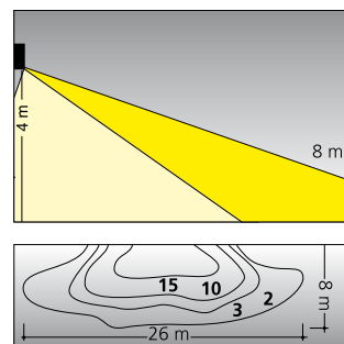
Вертикальный монтаж
