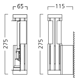
Настенный светильник Tube 9Вт
