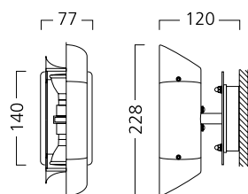
Настенный Trend двусторонний 2x35Вт
