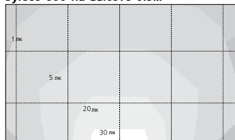
Syleos 600 на высоте 0.5м
