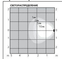
Верт. Hi-Spot ES50 50Вт
