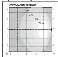
Горизонт. Lynx-D 18Вт
