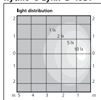
Rytmo C Lynx-D 18Вт
