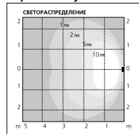
Вертикал. Lynx-D 18Вт
