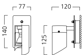
Настенный Trend односторонний 1x35Вт
