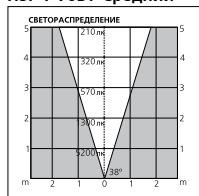
HSI-T 70Вт Средний
