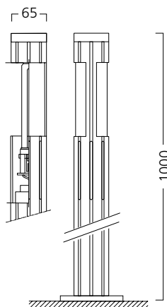
Столбик XL 11Вт
