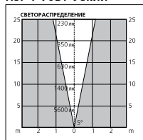
HSI-T 70Вт Узкий
