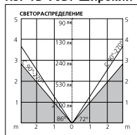
HSI-TD 70Вт Широкий
