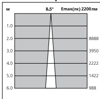
100Вт 8° Спот/ с антислеп. экраном
