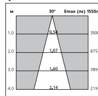
QPAR30 100Вт
