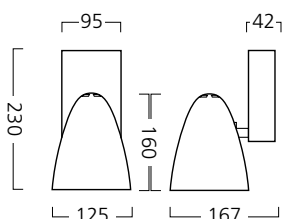
Punto Mono
