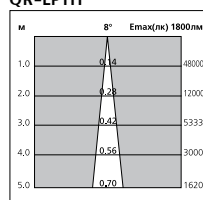
QR-LP111
