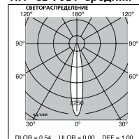
HIT-CE 70Вт Средняя
