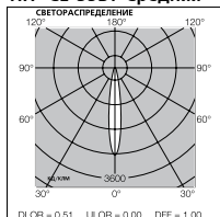
HIT-CE 35Вт Средняя
