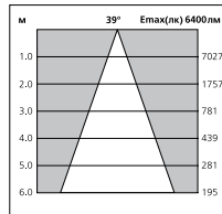
НЛТ-ТС-СЕ 70Вт 39°
