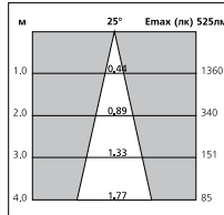
QPAR51 50Bт
