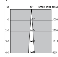
QPAR30 100Вт
