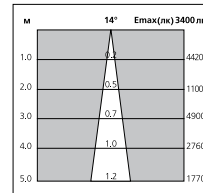
HIT 35Вт
