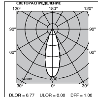
HIT-CE 70Вт Заливающ.
