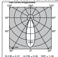
HIT-CE 35Вт Заливающ.
