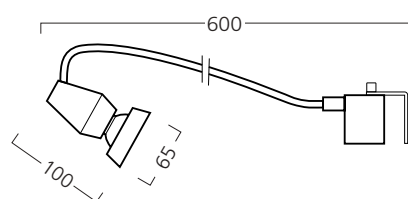
Display BriteSpot Двойная изоляция, заземление обеспечивают ЭМС фильтр.
