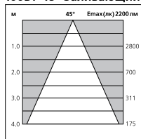
100Вт 45° Заливающий
