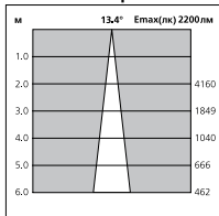
100Вт 14° Спот/ с антислеп. экраном
