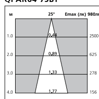
QPAR64 75Вт
