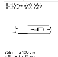
СДМ-ТС/СМЛ-ТС
