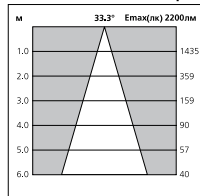
100Вт 34° Заливающий
