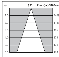
НЛТ-ТС-СЕ 35Вт 37°
