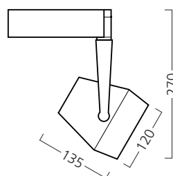
XL HIT/CMI-TC HIT/CMI-T Размеры бокса ПРА: 175x105x50мм
