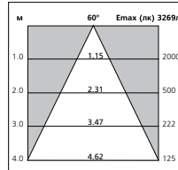
HIPAR51 35Вт
