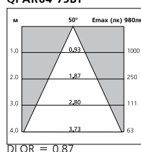
QPAR64 75Вт
