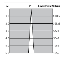
100Вт 7° Спот
