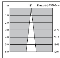
150Вт 15° Спот
