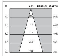
HIT 70Вт
