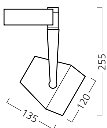
XL CMI-T 35W Размеры бокса ПРА: 125x75x40мм
