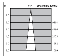
35Вт 11° Спот
