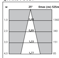
QPAR51 50Вт
