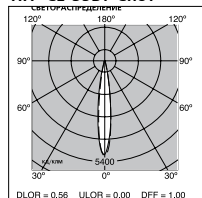
HIT-CE 35Вт Спот
