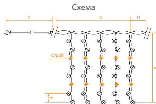
Последовательное подключение
