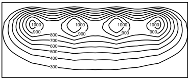
Isolux Diagram(lx)
