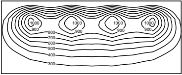
Isolux Diagram(lx)
